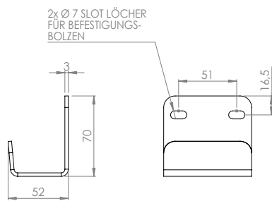
DETAILS DER „J“-WANDHALTERUNG
